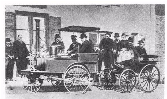
L'AUTOMOBILE A VAPEUR DE VIROT, CONSTRUITE DANS LES ATELIERS DE L'ECL (1884).
